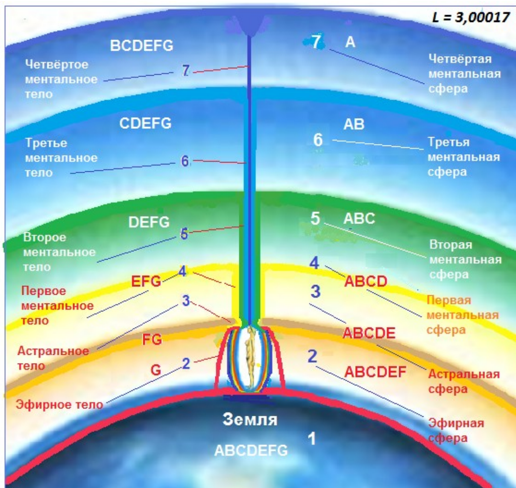
Рис.1. Связь тонких тел сущности со сферами Земли
