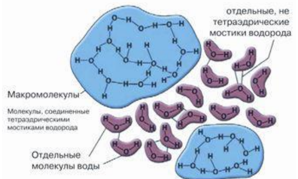
Рис.2. Некоторые структурные объединения молекул воды.
