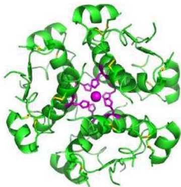
Рис. 10. Структура инсулина
