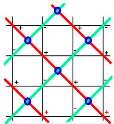
Рис. 3. Магнитные линии
