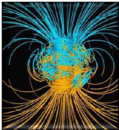
Рис. 5. Силовые линии магнитного поля
