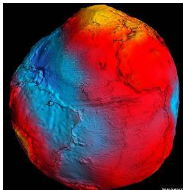
Рис. 2. Геоид Истинная форма Земли
