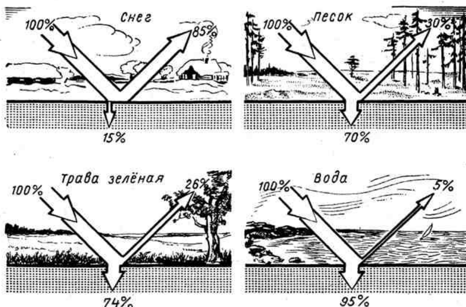
Альbedo различных видов земной поверхности
