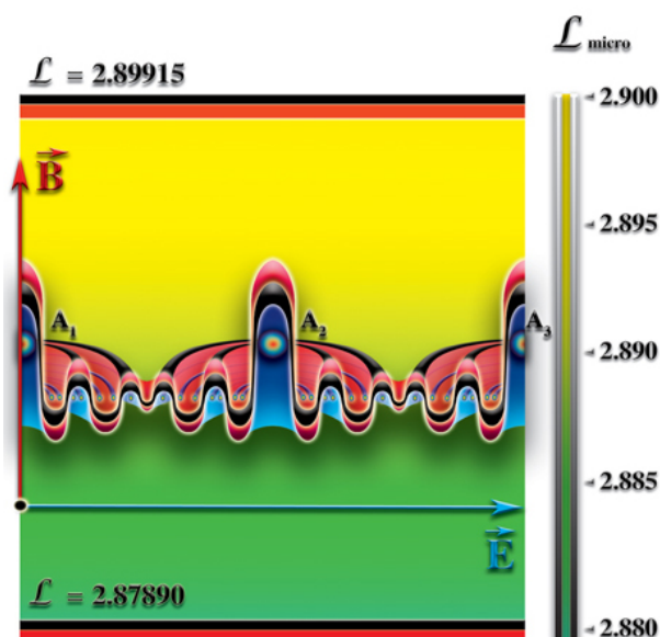
Электрическое (E) и магнитное (B) поля как следствие перепада мерности
