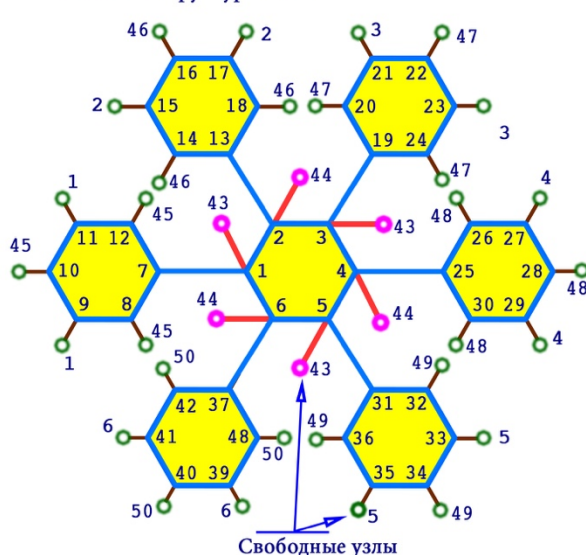
Бензольная структура золота
