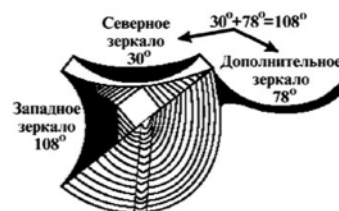
Схема основной Пирамиды тибетского комплекса – горы Кайлас (вид сверху). Показаны три гигантских
