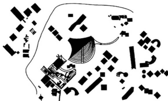
Схема расположения Пирамид комплекса Кайласа в Тибете
