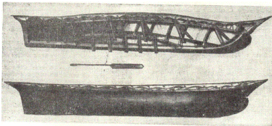
Разрез и общий вид лодки
